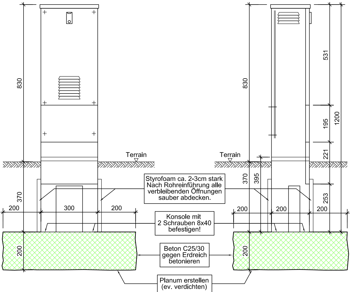
Längsschnitt
