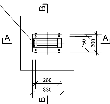
Grundriss
