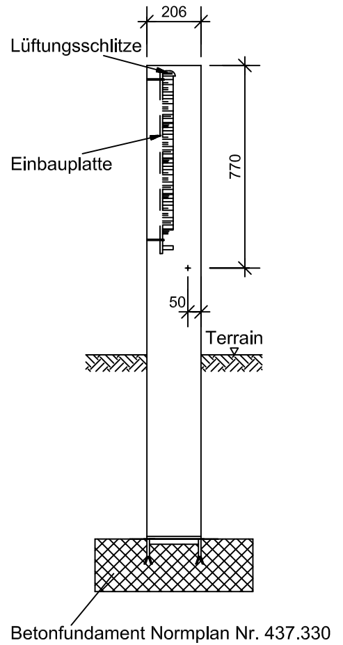
Schnitt B - B
