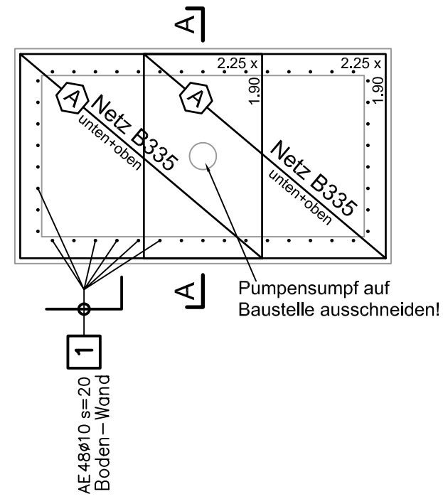
Grundriss 1:50 Armierung Boden
