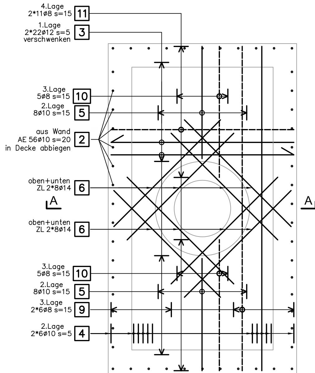
Grundriss 1:25 Armierung Decke
