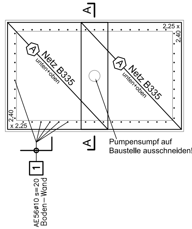
Grundriss 1:50 Armierung Boden
