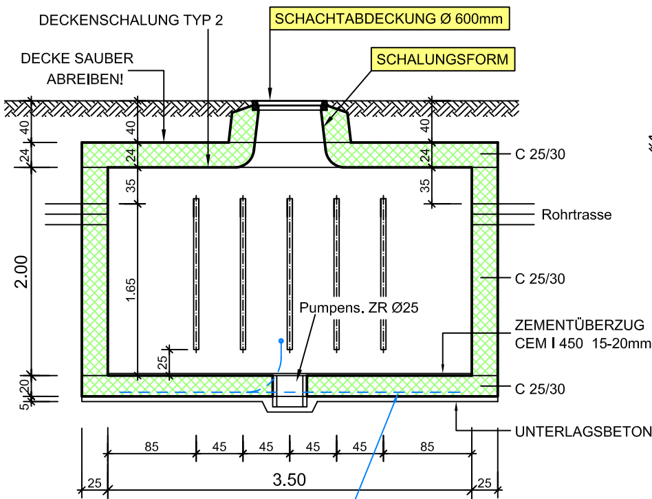
Längsschnitt 1:50
