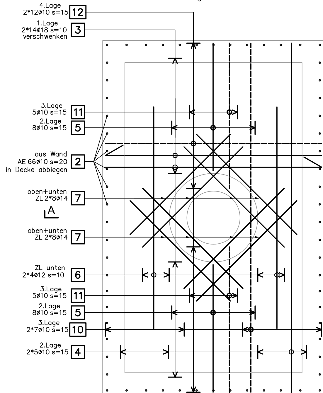
Grundriss 1:25 Armierung Decke
