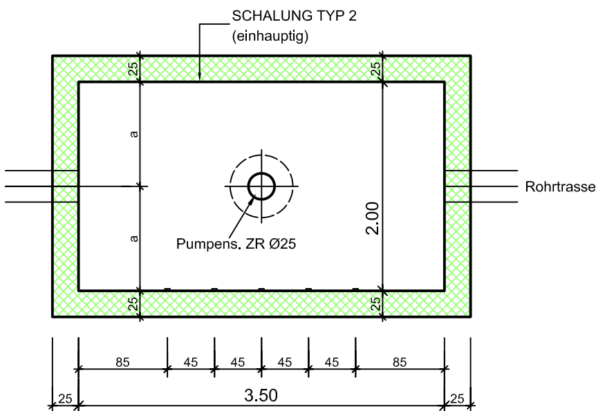
Grundriss 1:50
